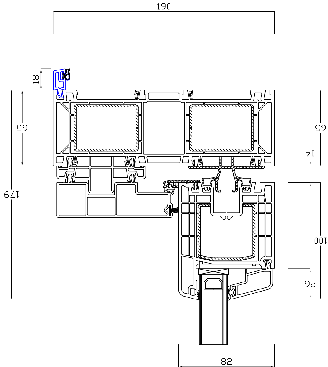
Detail: T9-F05-BD met aanslag Schaal 1:2
